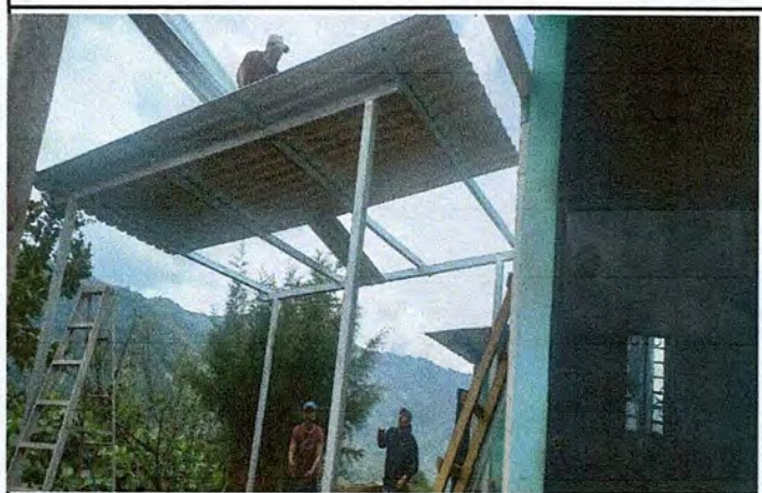
Foto 4: AVANCE TIPO PORTICO METÁLICO E INSTALACIÓN DE LÁMINA TROQUELADA CALIBRE
